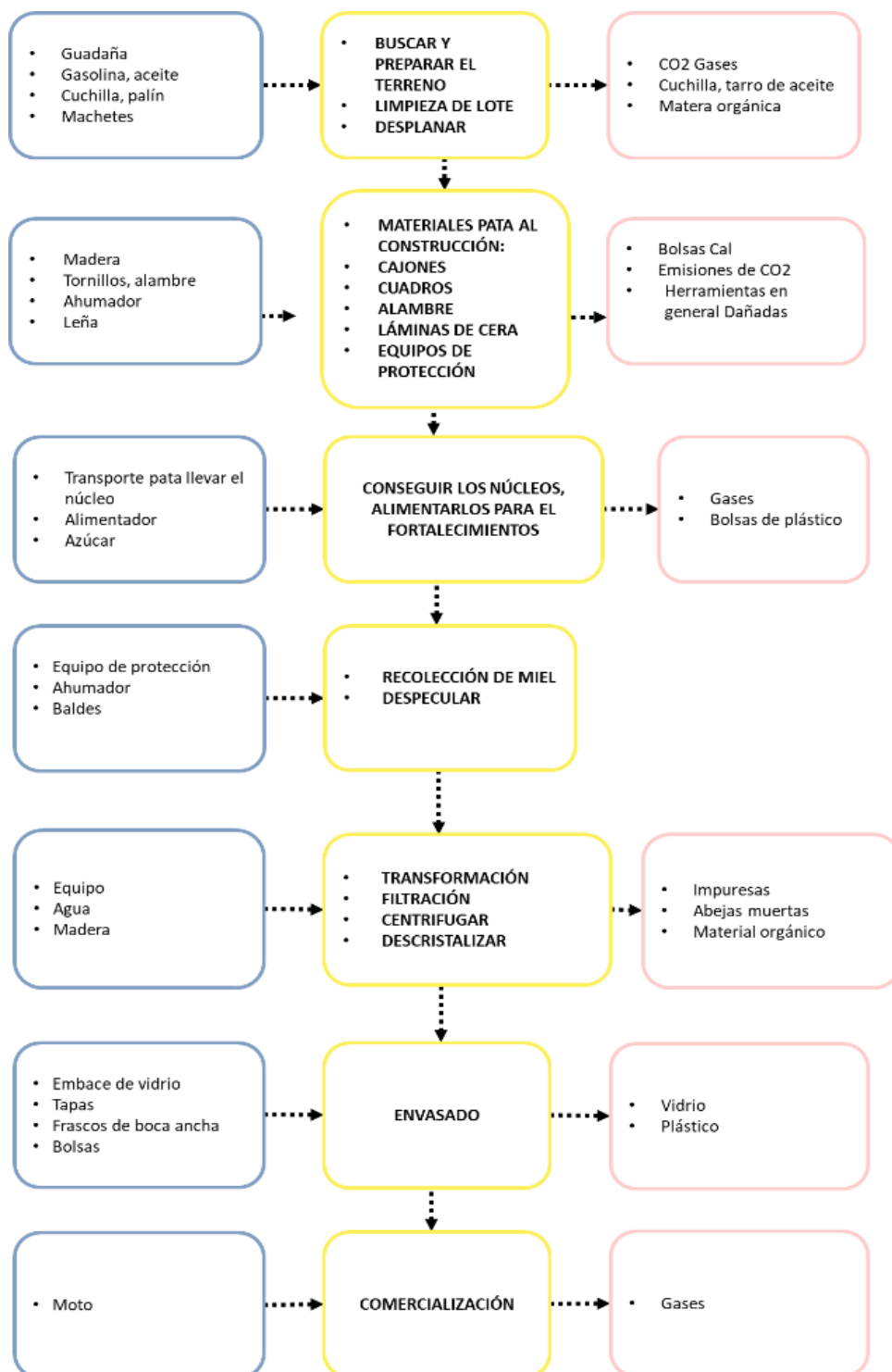
Figura 2 Diagrama de proceso producción Apícola.
