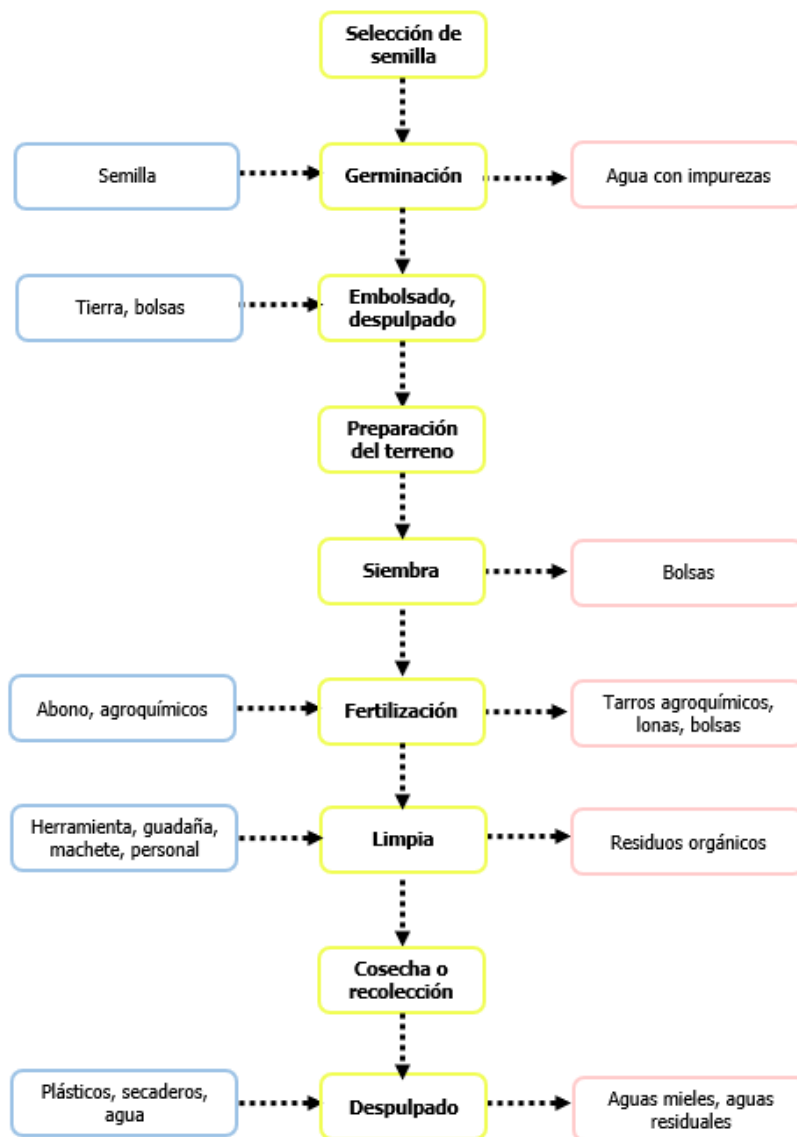
Figura 2 Diagrama de proceso producción de café
