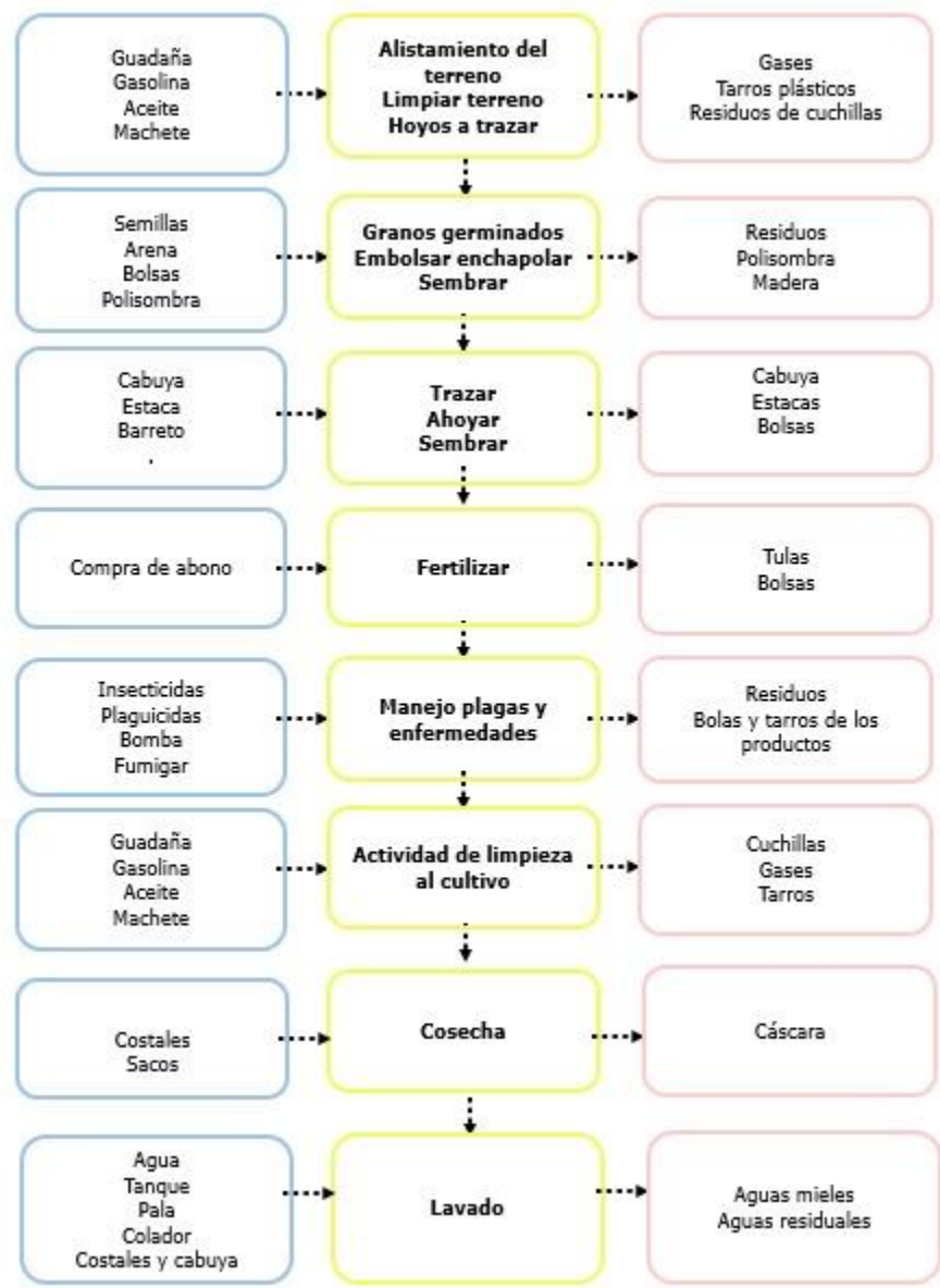
Figura 2 Diagrama de proceso producción de café
