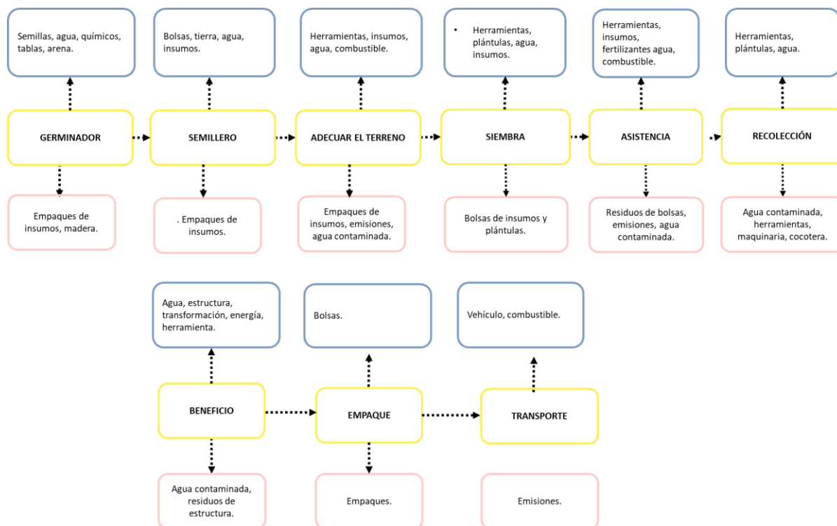
Figura 2 Diagrama de proceso producción de café.
