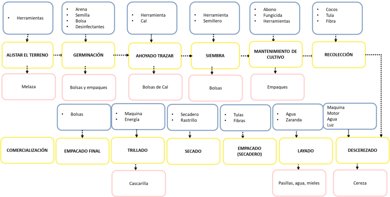
Figura 2 Diagrama de proceso producción de café.
