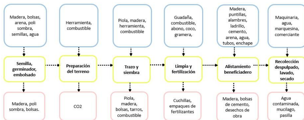
Figura 2 Diagrama de proceso producción de café
