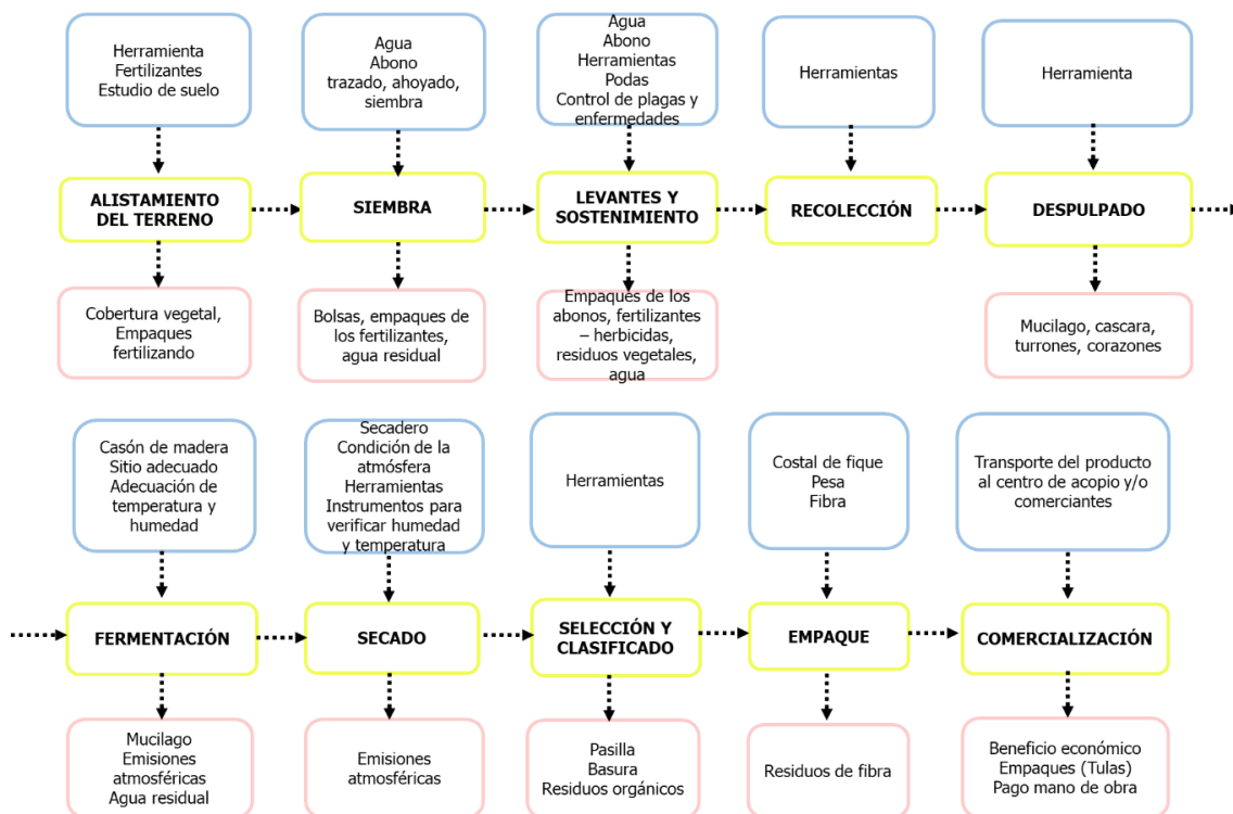
Figura 2 Diagrama de proceso producción de cacao.
